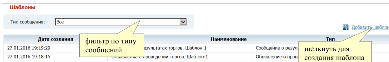
Рис. 52. Страница «Шаблоны».
