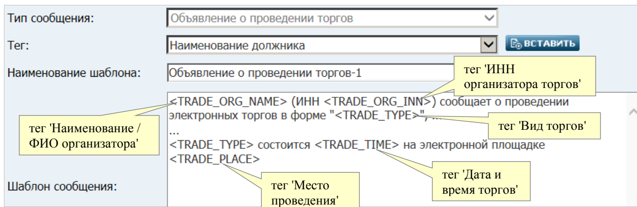
Рис. 54. Пример тегов, вставленных в шаблон сообщения.
