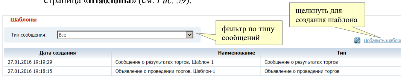
Рис. 59. Страница «Шаблоны».
