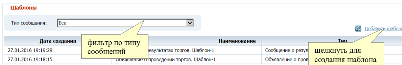
Рис. 61. Страница «Шаблоны».
