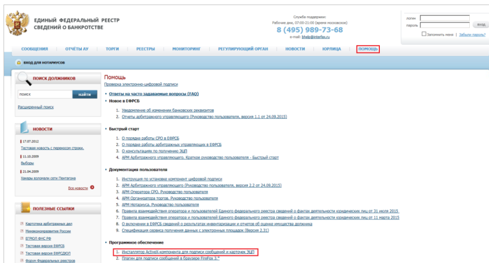
Рис. 1. Страница «Помощь».
