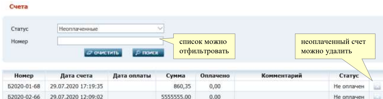
Рис. 62. Страница «Счета».
