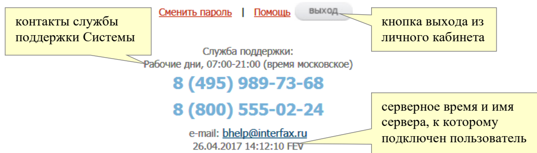
Рис. 4. Информационно-функциональный блок.
