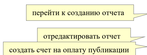
Рис. 12. Страница «Отчеты».
