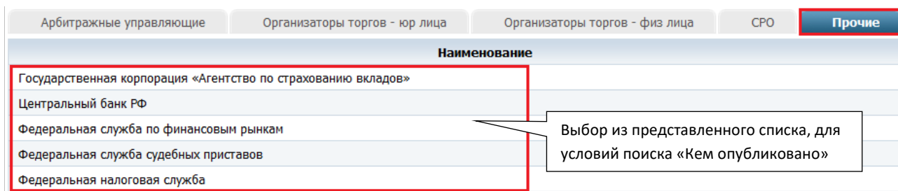
Рис. 12. Вкладка «Прочие».
