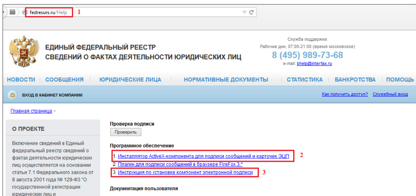
Рис. 1. Страница «Помощь».
