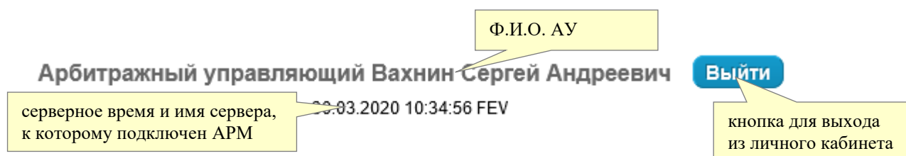
Рис. 6. Информационно-функциональный блок.
