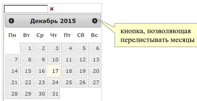
Рис. 41. Встроенный календарь.
