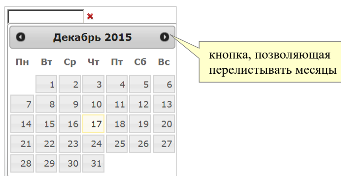
Рис. 87. Встроенный календарь.
