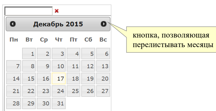
Рис. 44. Встроенный календарь.
