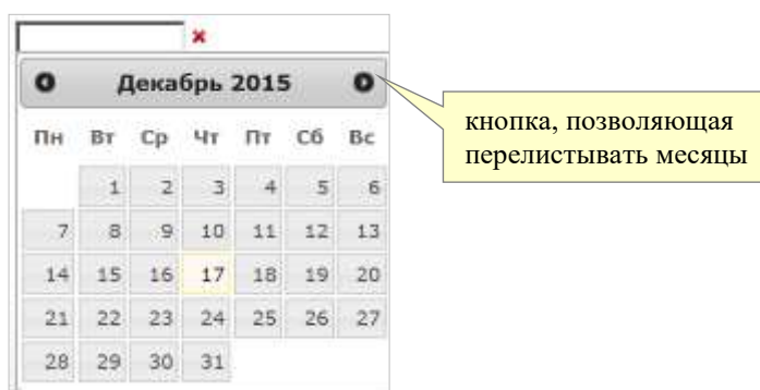
Рис. 108. Встроенный календарь.
