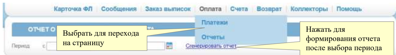
Рис. 87. Страница «Отчеты».
