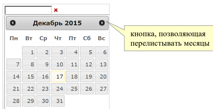
Рис. 108. Встроенный календарь.
