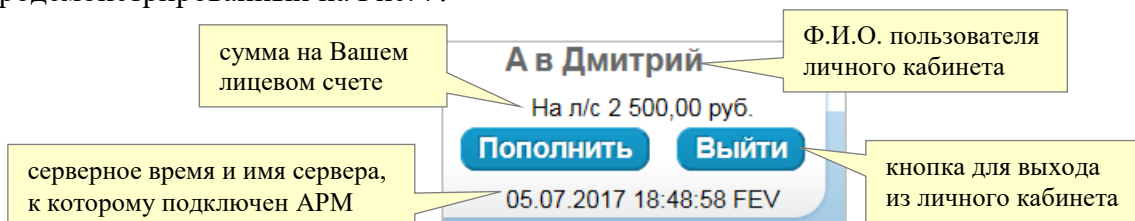
Рис. 7. Информационно-функциональный блок.
