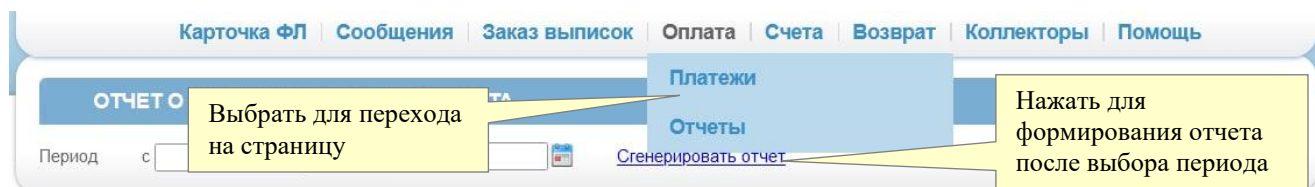
Рис. 87. Страница «Отчеты».
