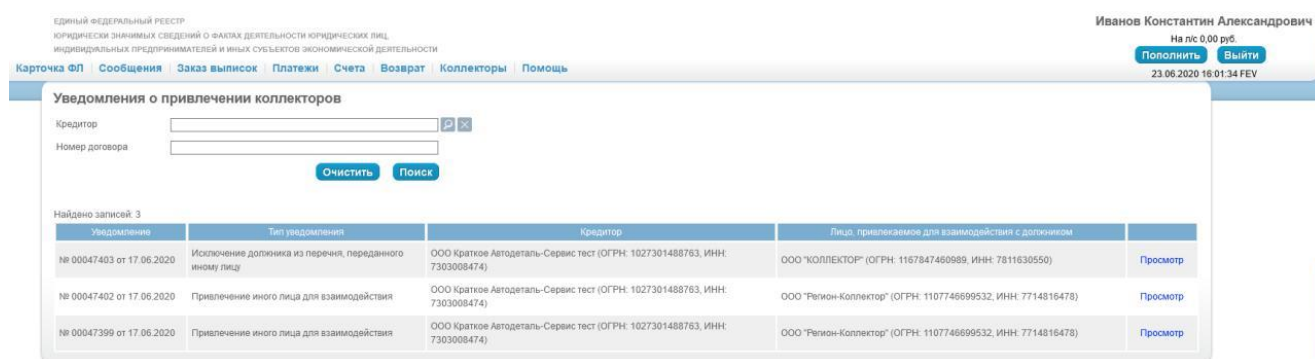
Рис. 101. Страница «Коллекторы».
