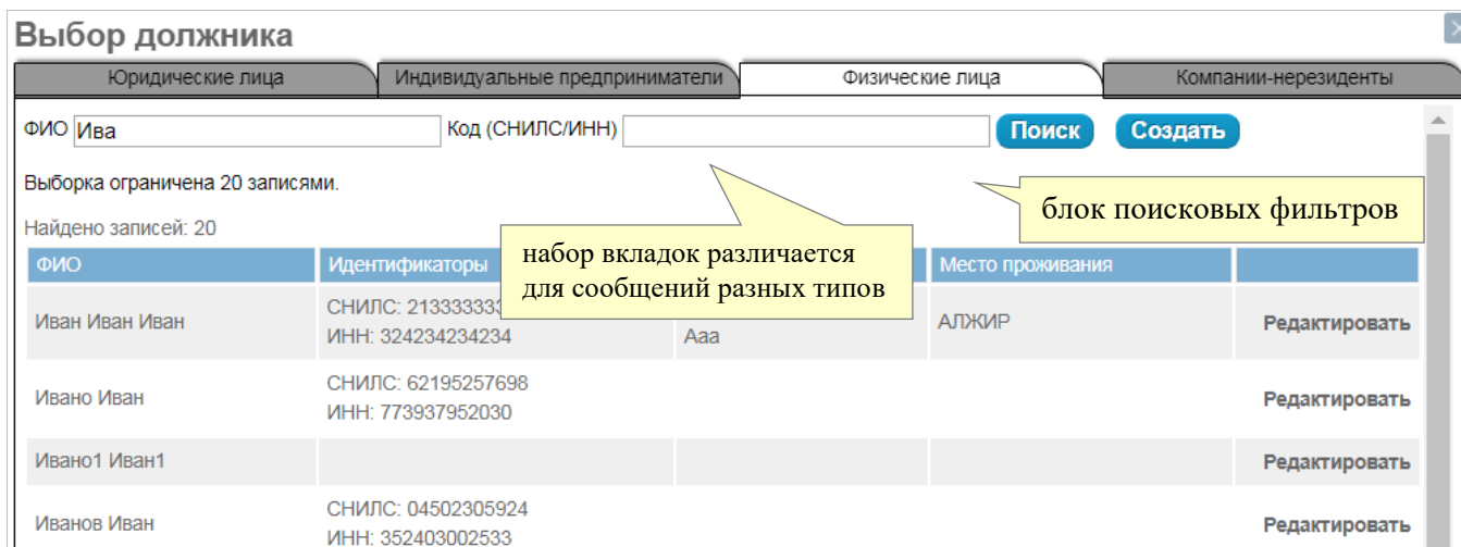
Рис. 44. Окно для выбора участника сообщения.
