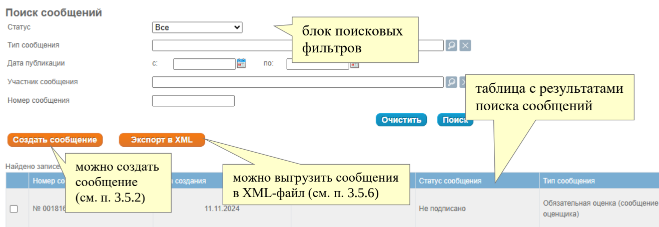
Рис. 11. Страница «Сообщения»
