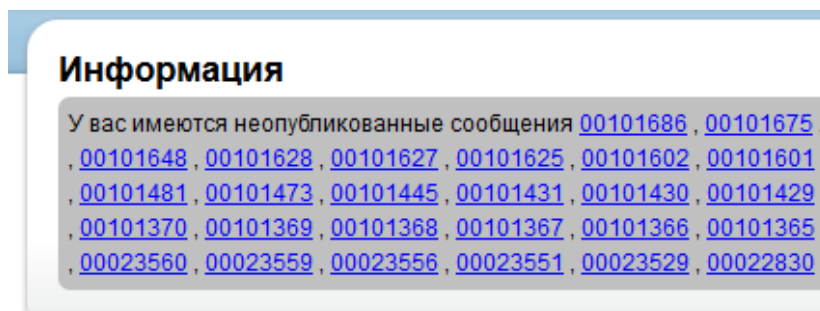
Рис. 10. Страница «Информация»
