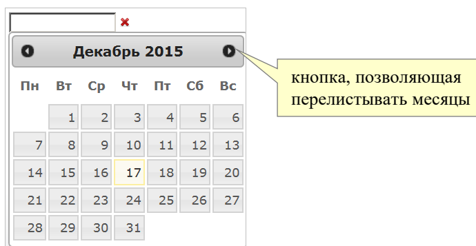
Рис. 49. Встроенный календарь.
