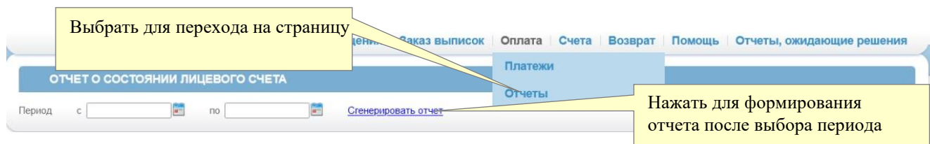
Рис. 30. Страница «Отчеты».
