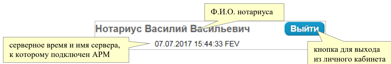
Рис. 5. Информационно-функциональный блок.
