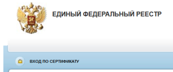
Рис. 2. Авторизация пользователя.
