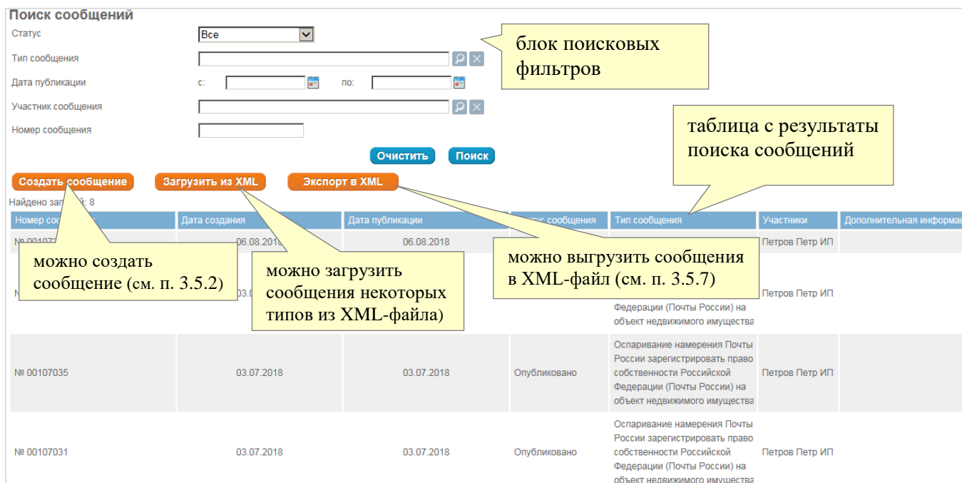
Рис. 16. Страница «Сообщения»
