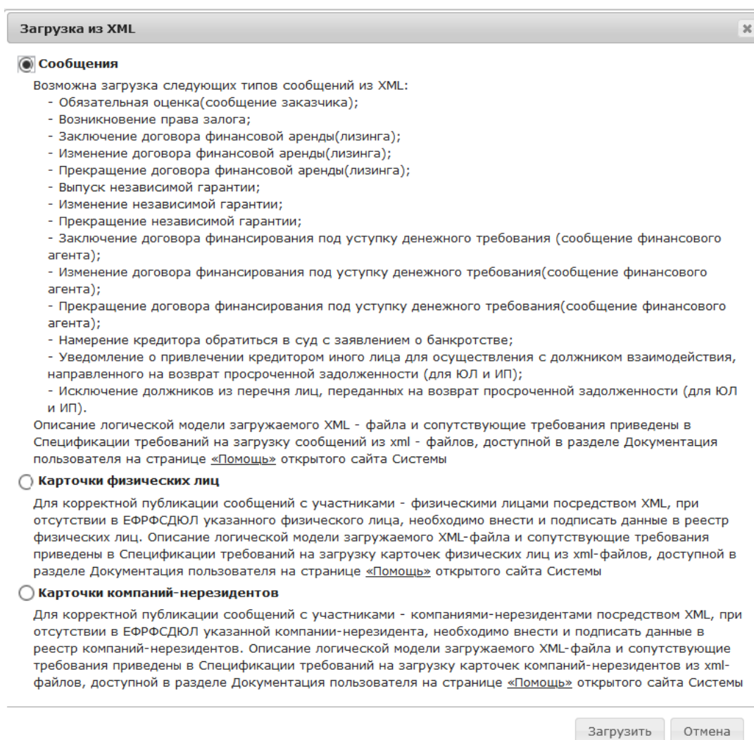
Рис. 98. Окно «Загрузка из XML».
