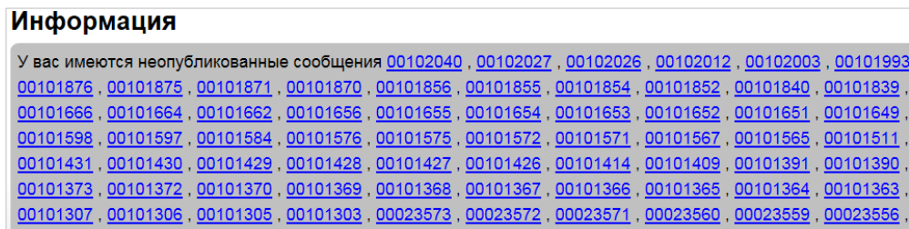
Рис. 18. Страница «Информация».
