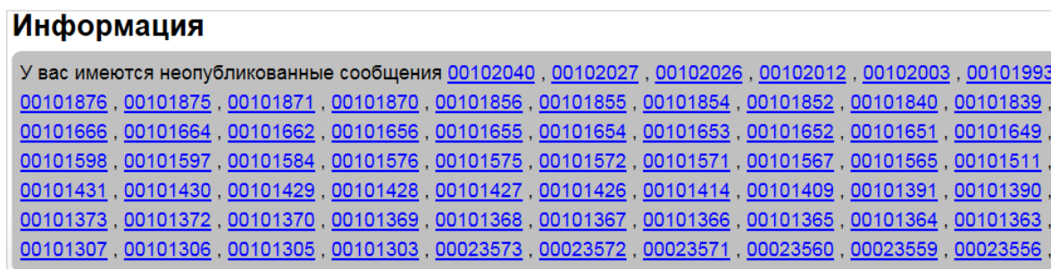
Рис. 18. Страница «Информация».
