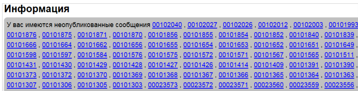
Рис. 22. Страница «Информация».
