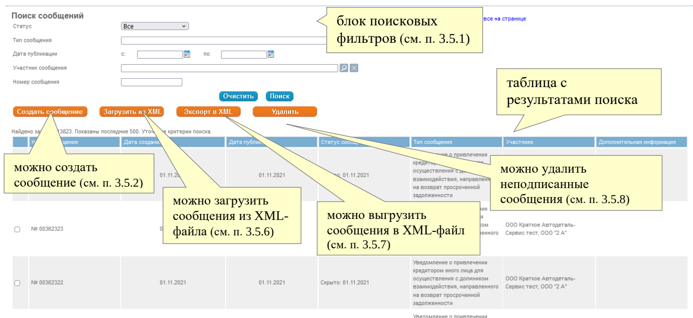
Рис. 23. Страница «Сообщения».
