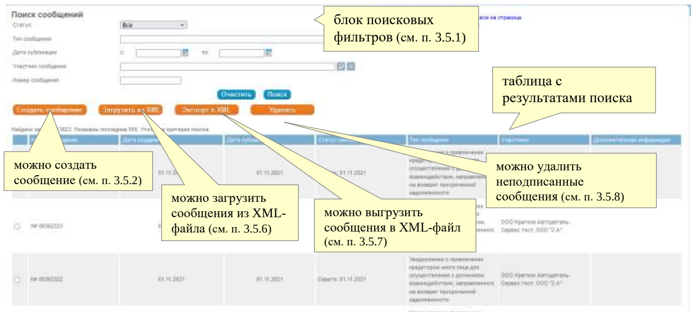
Рис. 19. Страница «Сообщения».
