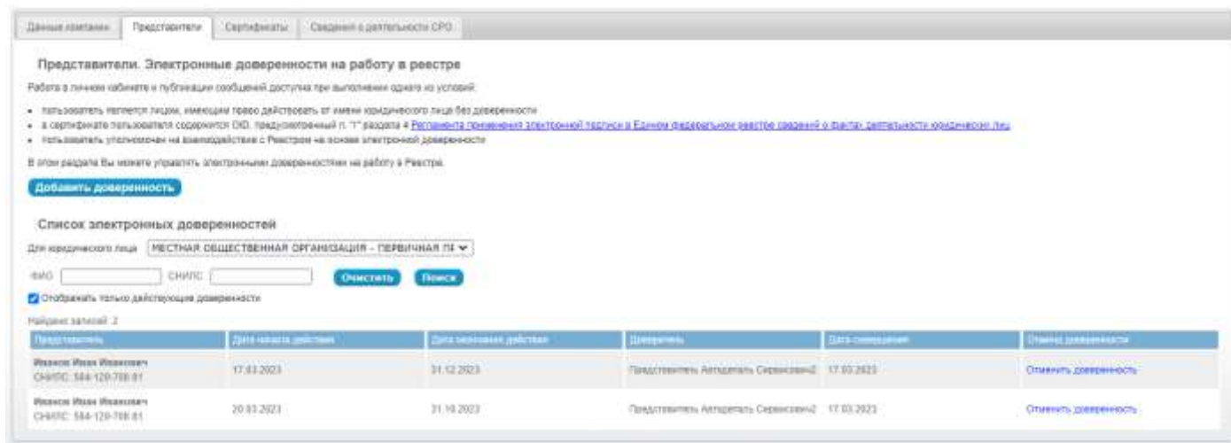
Рис. 10. Вкладка «Представители».
