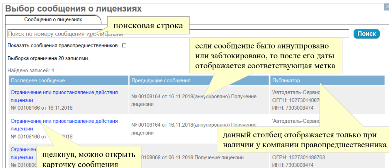
Рис. 206. Окно «Выбор сообщений о лицензиях».
