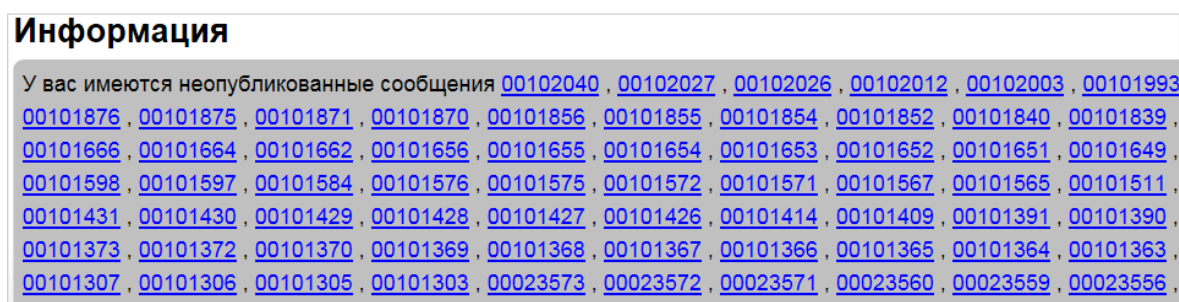
Рис. 20. Страница «Информация».
