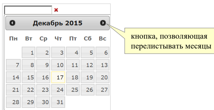
Рис. 76. Встроенный календарь.
