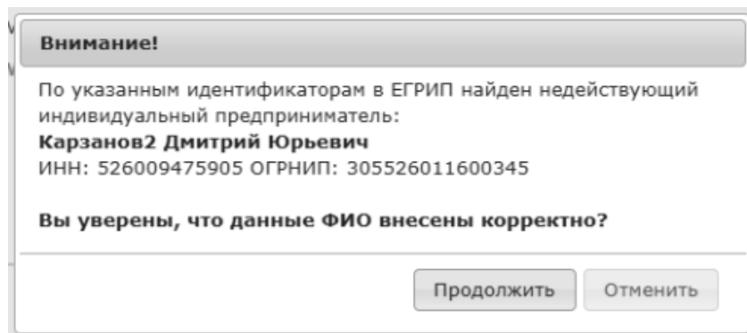
Рис. 182. Карточка создания физического лица (найдено совпадение по ИНН с недействующим ИП из реестра ИП )
