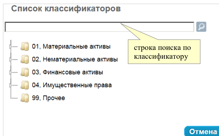
Рис. 183. Окно классификатора имущества
